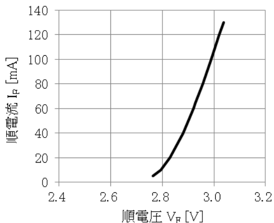
I_F - V_F ( T_a=25^\circ\text{C} )
