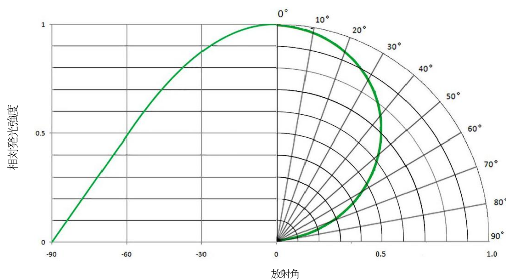
放射角-相対強度 (光束) 特性
