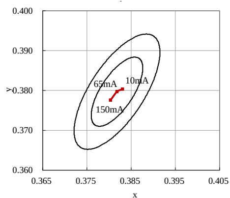
色度 - I_F ( T_a=25^\circ\text{C} )
