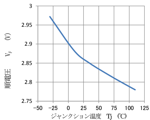
V_F - T_j ( I_F=65\text{mA} )
