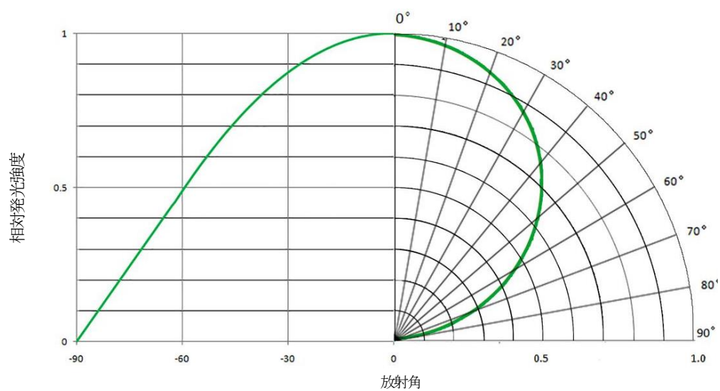
放射角-相対強度（光束）特性
