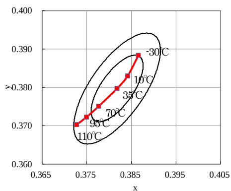
色度 - T_j ( I_F=65\text{mA} )
