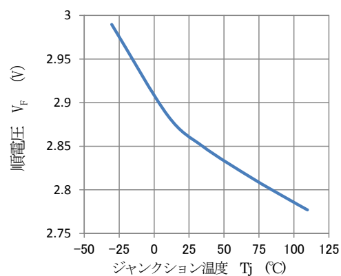
V_F - T_j ( I_F=65\text{mA} )
