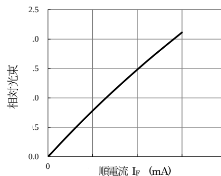
相対光束 - I_F ( T_a=25^\circ\text{C} )
