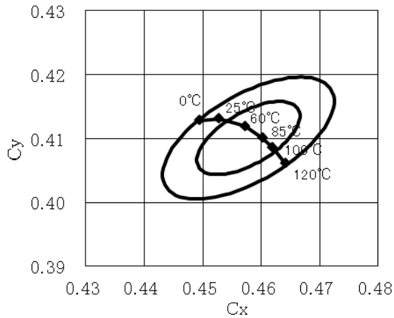
色度 - T_j ( I_F=65\text{mA} )
