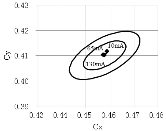
色度 - I_F ( T_a=25^\circ\text{C} )
