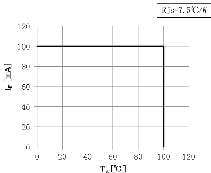
ディレーティング特性
