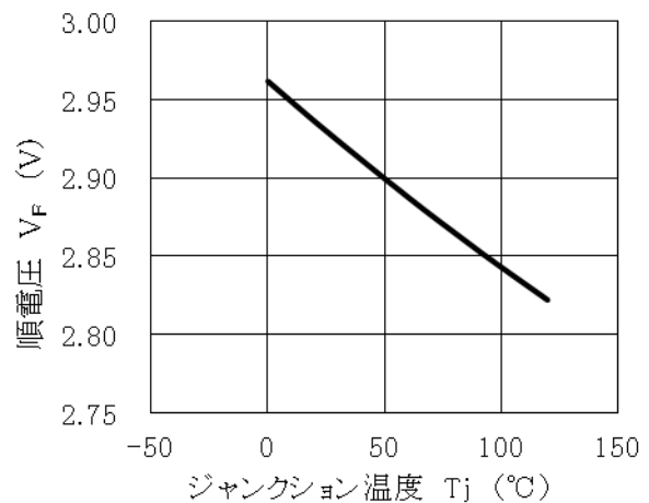
V_F - T_j ( I_F=65\text{mA} )
