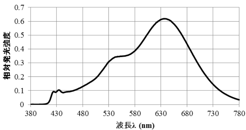
波長特性 (Ta=25°C, I F =65mA)
