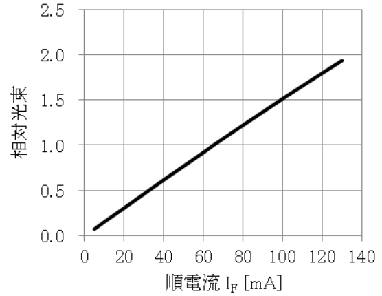
相対光束 - I_F ( T_a=25^\circ\text{C} )
