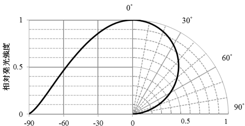
放射角-相対強度 (光束) 特性 (Ta=25°C, I F =65mA)
