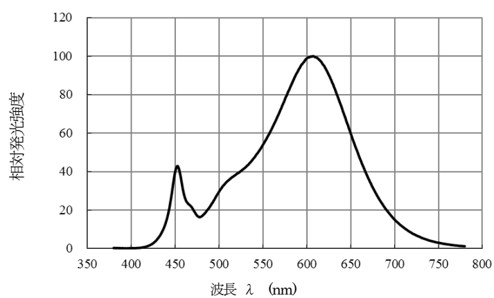
波長特性
