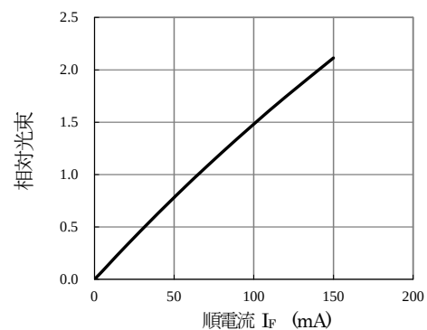
相対光束 - I_F ( T_a=25^\circ\text{C} )
