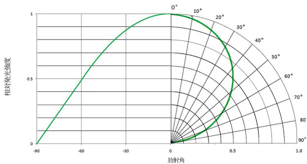
放射角-相対強度 (光束) 特性
