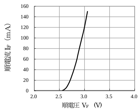
I_F - V_F ( T_a=25^\circ\text{C} )
