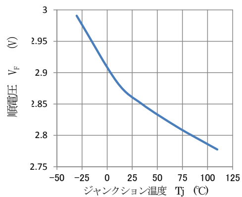
V_F - T_j ( I_F=65\text{mA} )
